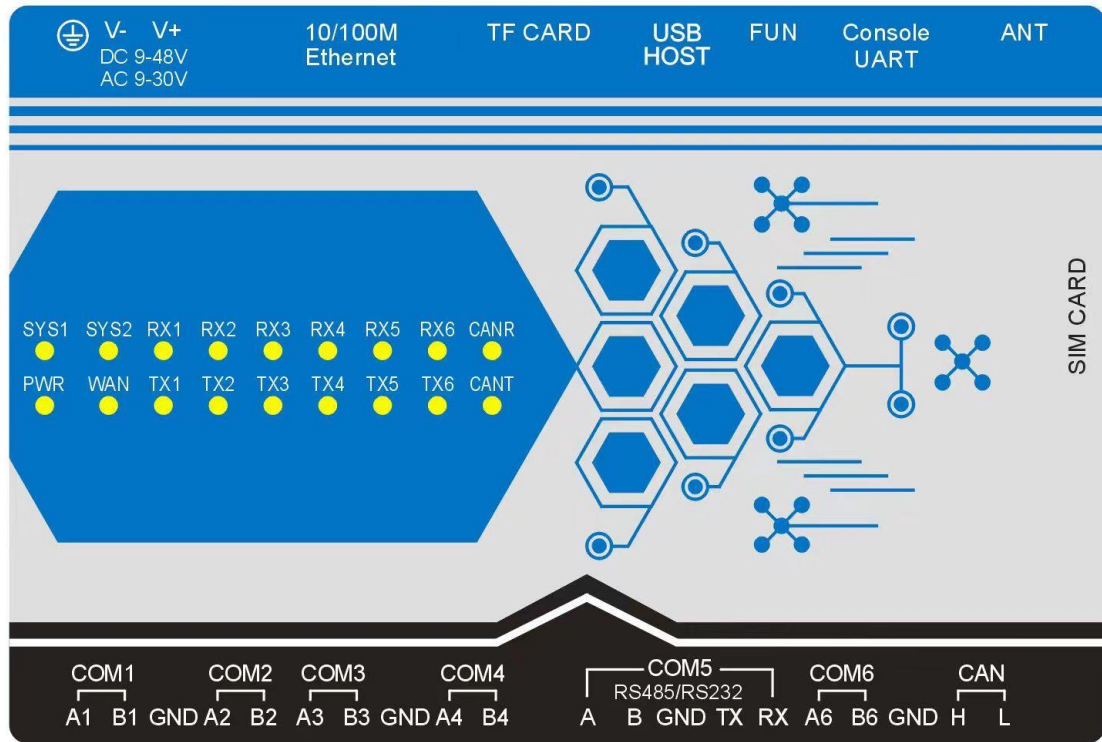
图 2.2.1 箱体正面图
